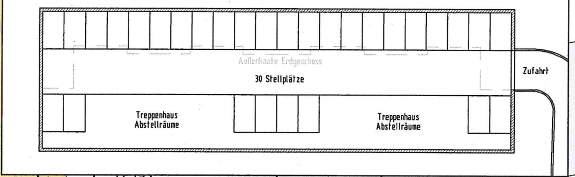
Tiefgaragengrundriss (Halbgeschoss)
